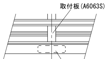
接続金具 (A5052 1.5t) ◇差込式
